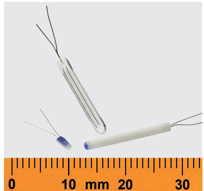
Fig. a sinistra: resistenza di misura a film sottile (con isolante)
