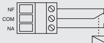
Relé 2 (opção)
