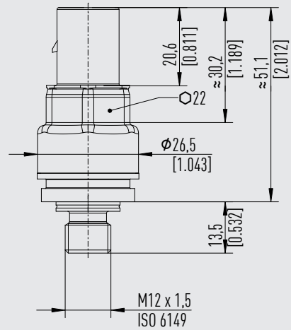
VW Stecker, Code I, 4-polig, 2-reihig
