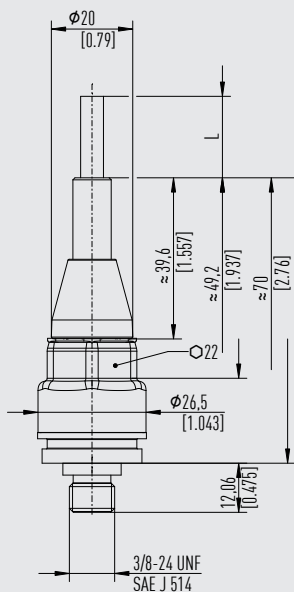
Kabelausgang, IP6K9K, 2- oder 3-Leiter
