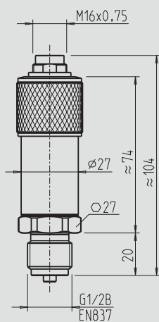
com M16 x 0,75 conector circular
